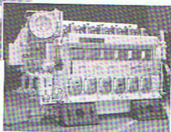
Motor 6R22MD-D de 1050 BHP a 900 RPM
