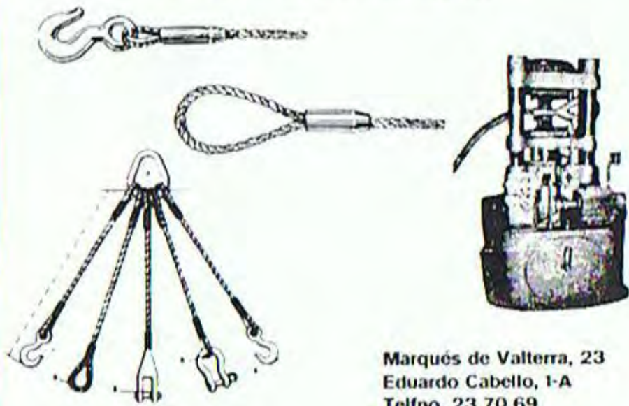
PRENSA DE 500 Tm. PARA COLOCACION DE CASQUILLOS METALICOS A ESLINGAS Y MANIOBRAS DE PESCA COLOCACION DE TERMINALES POR MEDIACION DE FUNDICION DE CINZ ELECTROLITICO
