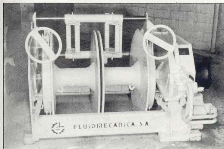
MAQUINILLAS DE ARRASTRE
