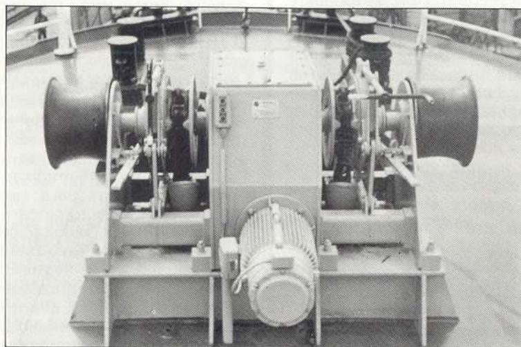
MOLINETES DE ANCLA
