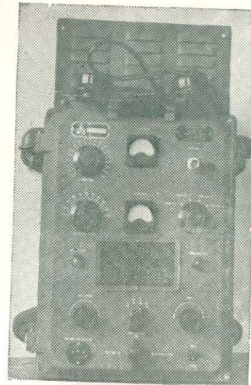
Radiotelefonía Marola II-A
