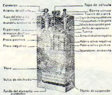
Corte a través de un elemento NIFE
